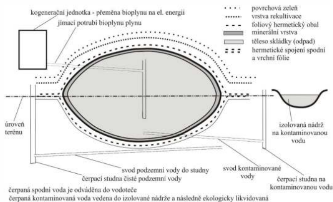
obr. č. 1 Zjednocené schéma řezu skládky
