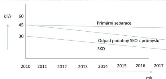
Obr. 1 Předpokládaný vývoj SKO v plánech odpadového hospodářství
